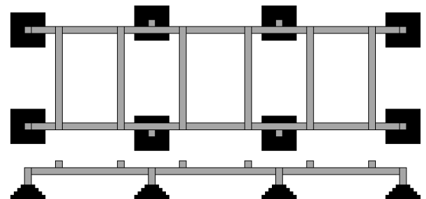
FXB/FXU-Frame
